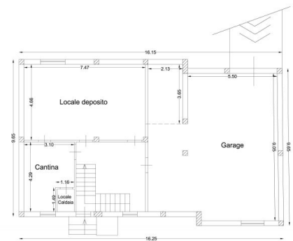
PIANTA CANTINATO
