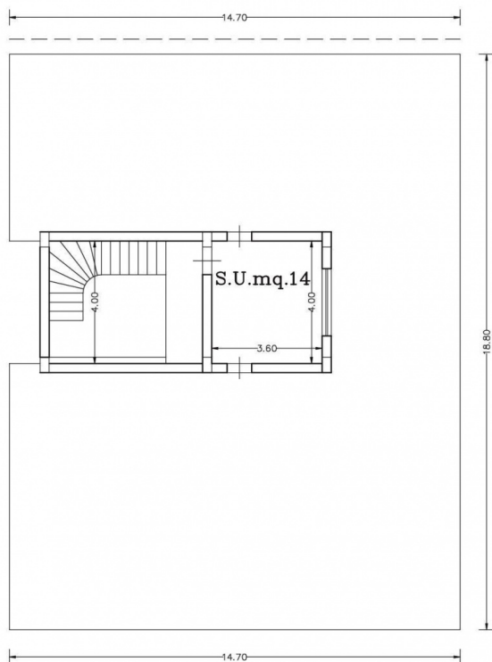
PIANTA PIANO PRIMO rapp. 1:100
