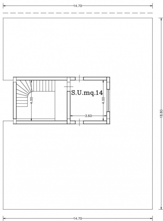
PIANTA PIANO PRIMO rapp. 1:100
