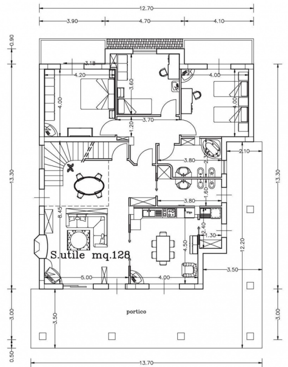
PIANTA PIANO RIALZATO rapp. 1:100
